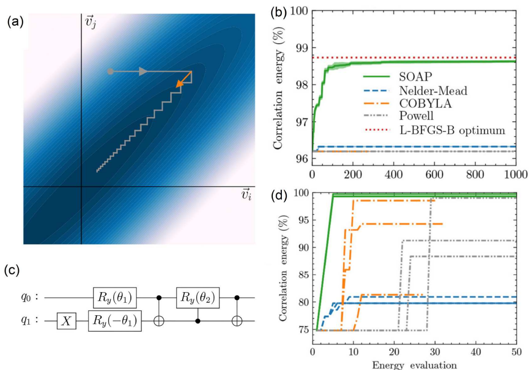
图 5 SOAP方法及其应用. (a) 当Hessian矩阵中存在较大的非对角元素时, 顺序优化方法的优化轨迹示意图. 传统的顺序优化方法从灰点开始, 然后沿着灰线继续进行. SOAP识别了一个更优的平均方向, 用橙色箭头标记, 显著加速了收敛 [27] . (b) SOAP与其他基于噪声模拟的无梯度优化方法的收敛速度对比. 量子噪声被建模为对测量能量的高斯噪声, 其标准偏差为1 mH. 与5个独立轨迹的标准偏差用阴影区域表示. 红色虚线是基于无噪声仿真的L-BFGS-B方法的最优值. 测试体系为N 2 分子 [27] . (c) 用于硬件实验的量子线路 [27] . (d) 基于QPU实验的SOAP与其他无梯度优化方法的收敛速度对比. 基准选取的是H 8 的(2e, 2e, 2o)活性空间近似的UCCSD计算, 对应于2个量子比特和2个线路参数. 对每种方法, 分别进行了3次独立的优化试验 [27]
